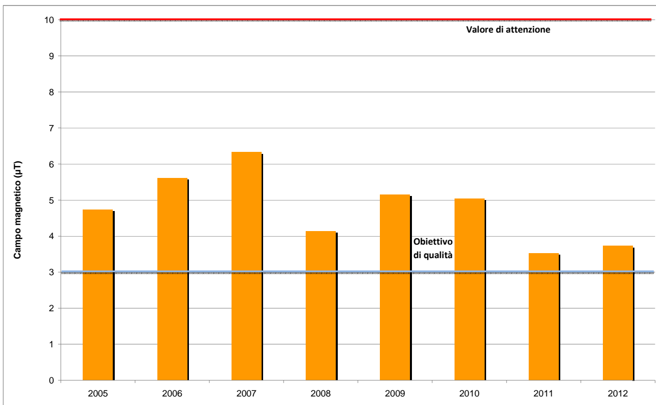
Grafico 6. Confronto massime medie giornaliere negli anni dell'induzione magnetica
