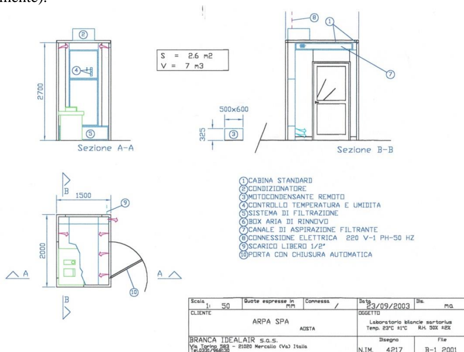
Schema della camera di pesata.
